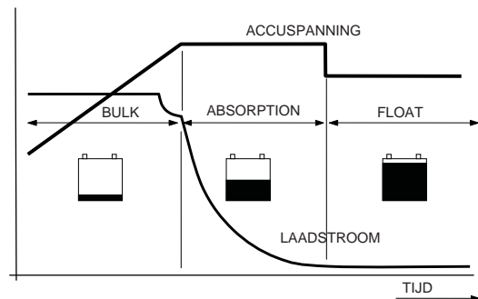
Afbeelding 3: Drietraps laadkarakteristiek
